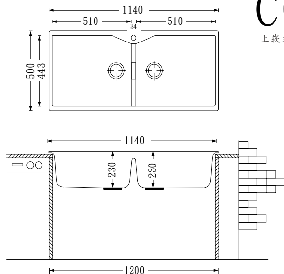
C02 P21 上嵌式 / 下嵌式
