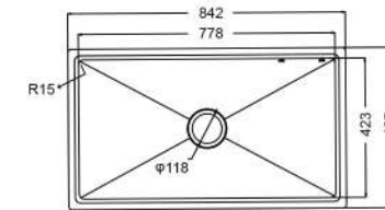
尺寸圖
