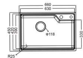
尺寸圖
