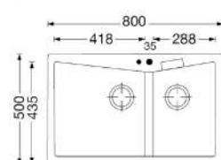
尺寸圖
