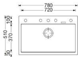
尺寸圖
