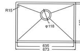
尺寸圖
