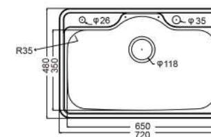
尺寸圖
