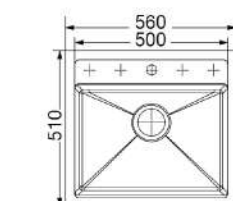
尺寸圖
