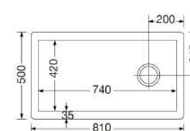
尺寸圖
